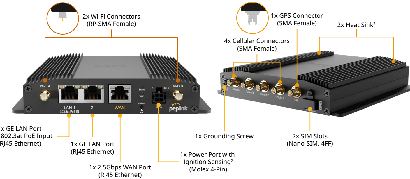
BR1 Pro 5G (HW3)
