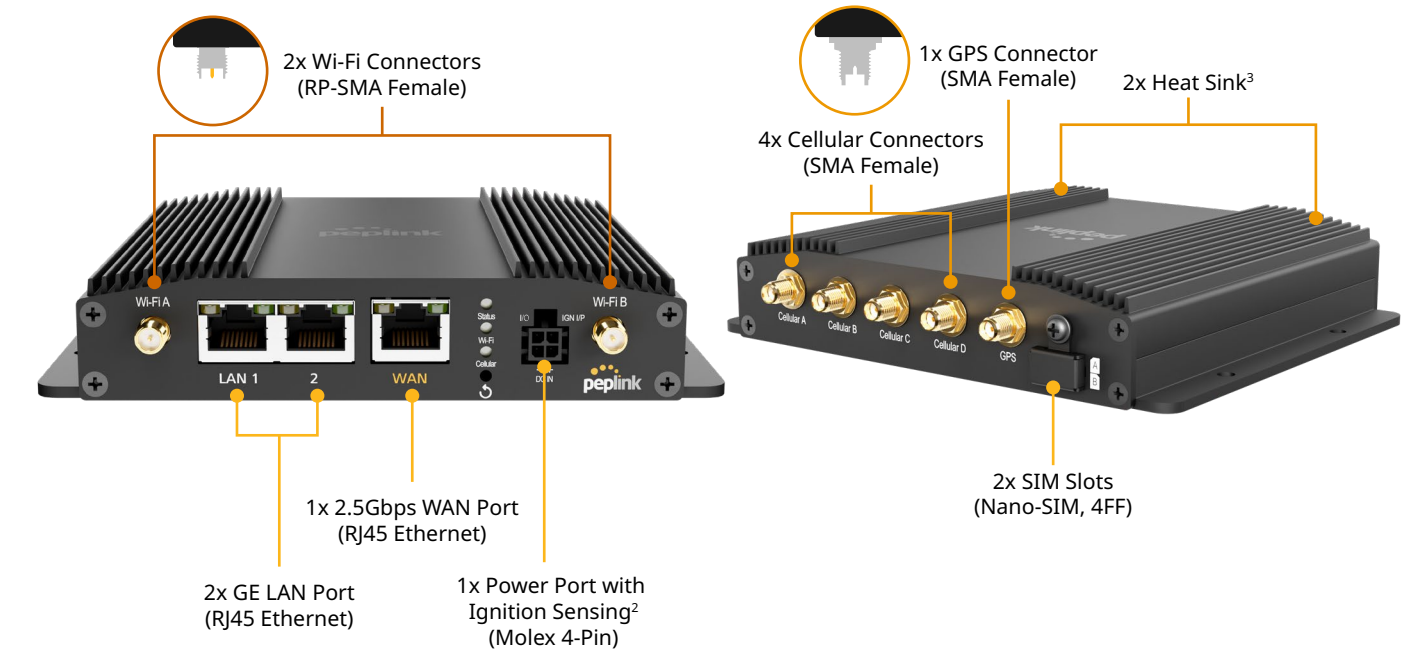
BR1 Pro 5G (HW2)
